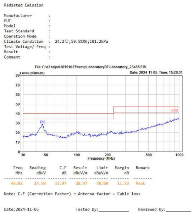
图 4-6 RE 测试垂直方向
