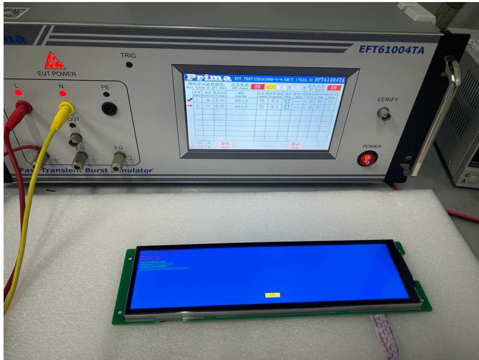
图 4-3 EFT 测试图
