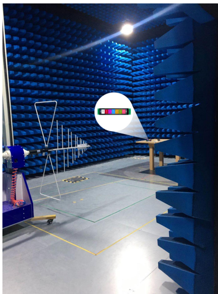
图 4-4 RE 测试图
